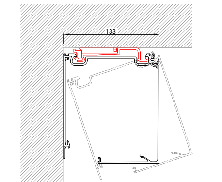
Supporto a molla
