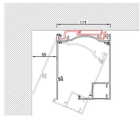
Supporto a molla per TEZWP120
