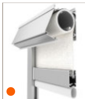
Cassonetto ispezionabile con guarnizioni anti insetto
