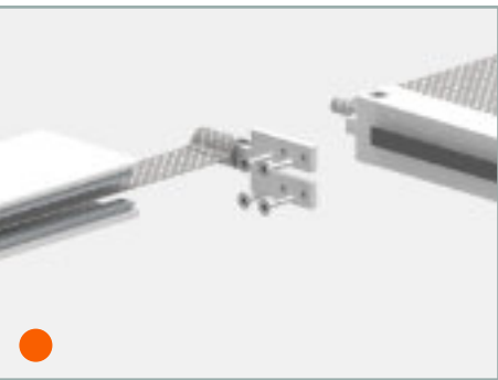
Fissaggio cinghia
