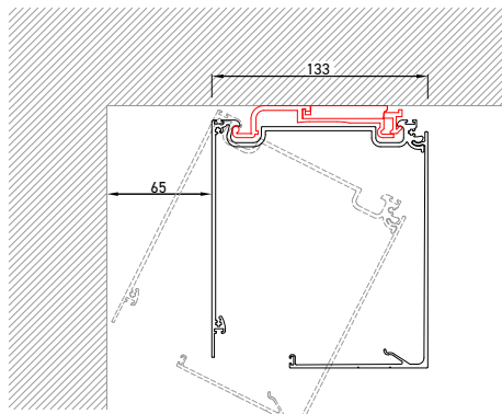
Supporto a molla per TEZWP130
