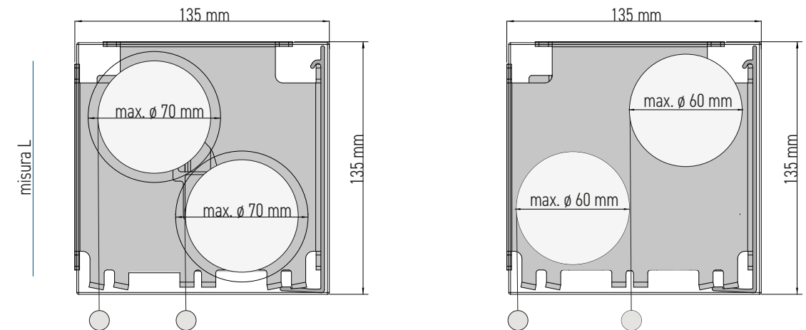
TENDA DOPPIA CON MANTOVANA
