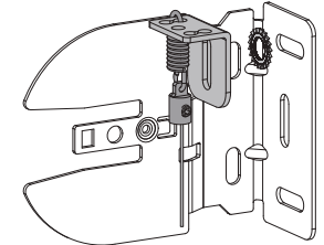
Attacco a muro
