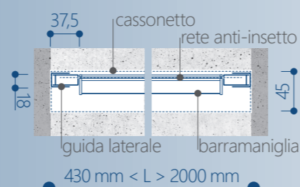
sezione orizzontale
