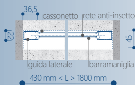
sezione orizzontale
