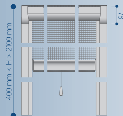
prospetto aperto
