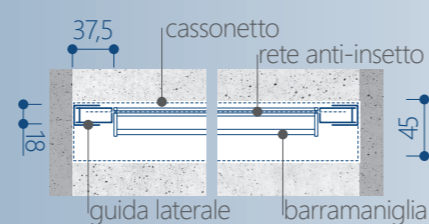
sezione orizzontale
