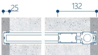
sezione orizzontale chiusa
