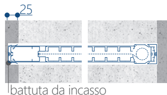
prospetto aperto
