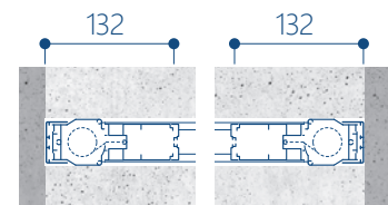
sezione orizzontale chiusa
