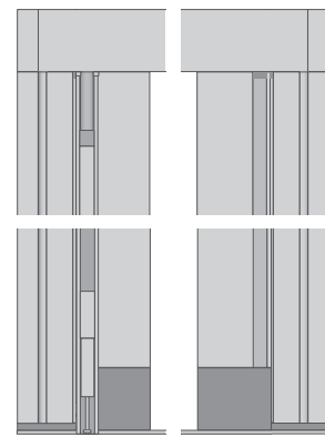
prospetto chiuso
