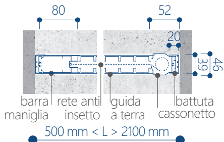
sezione orizzontale aperta
