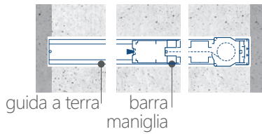
sezione orizzontale aperta
