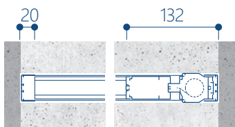
sezione orizzontale chiusa
