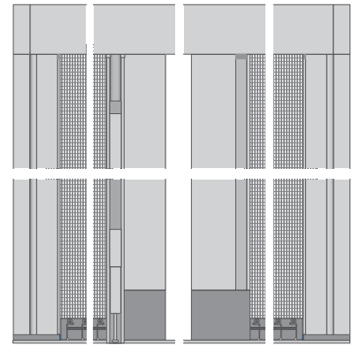
prospetto aperto
