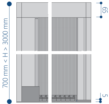
prospetto aperto
